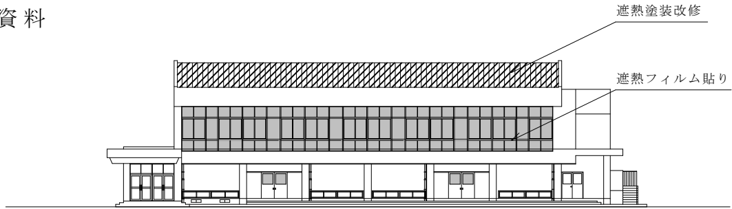
南立面図
