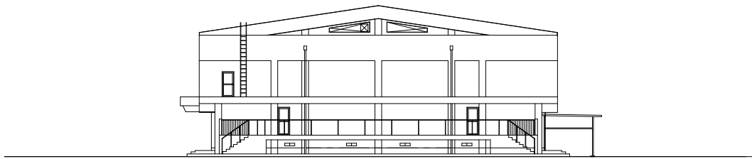
東立面図
