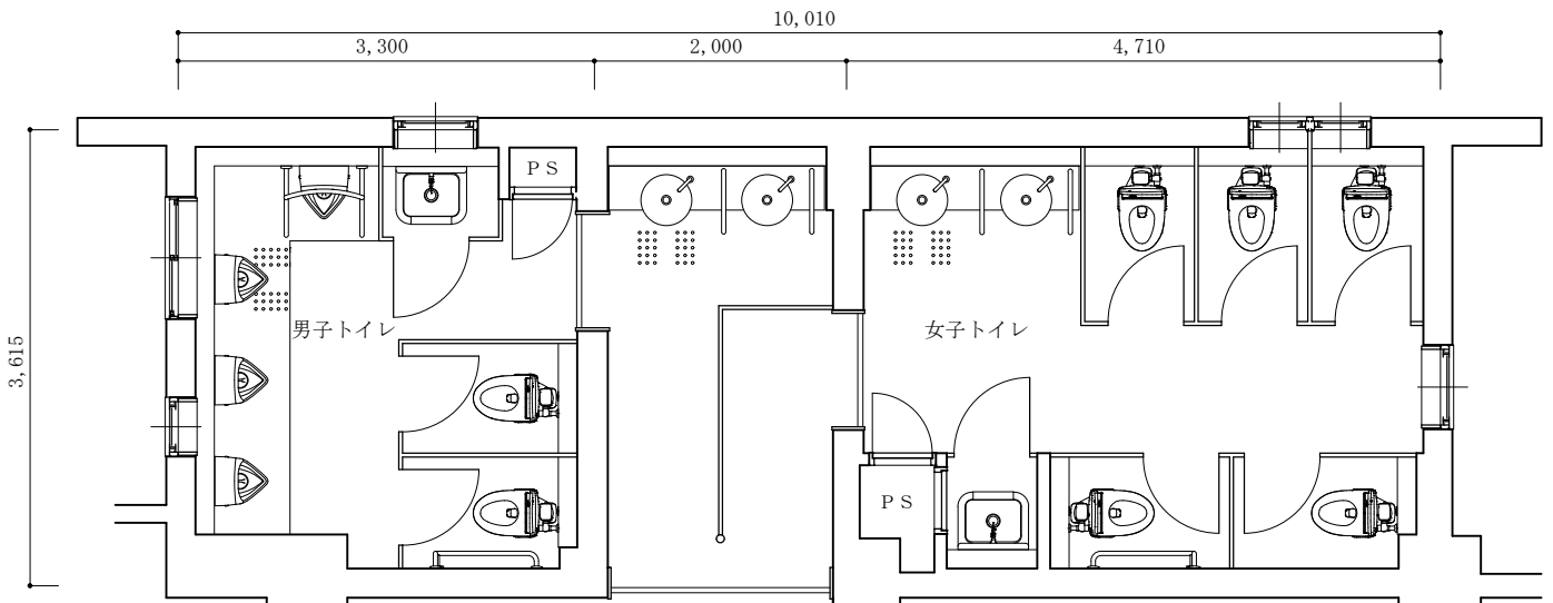
1階トイレ平面図
