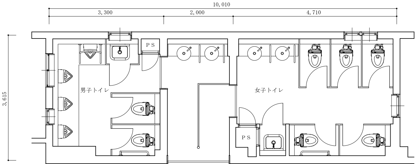
2階トイレ平面図
