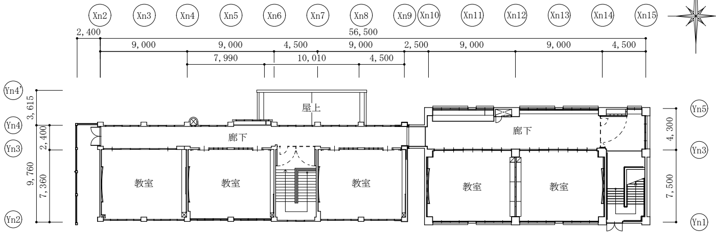
3階平面図
