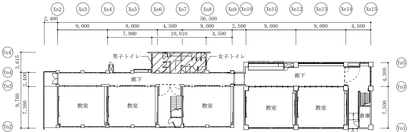
1階平面図
