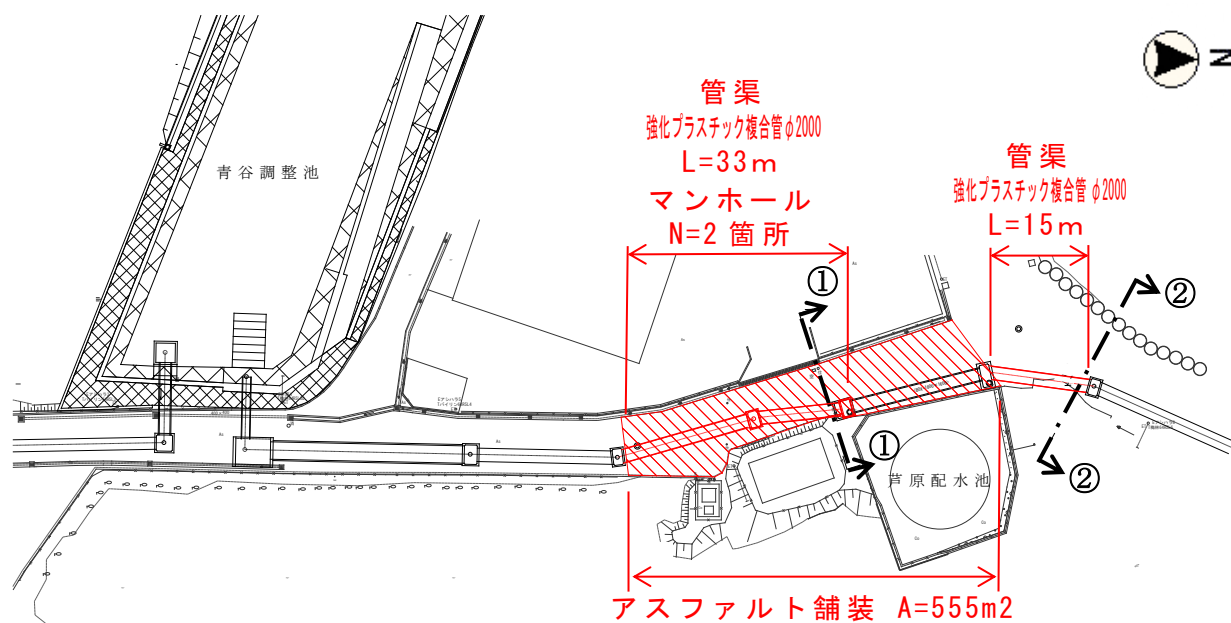
計画平面図
