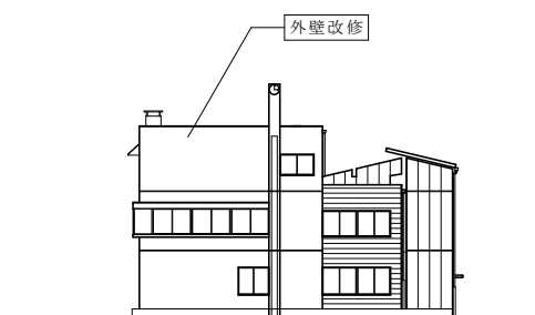
東面立面图
