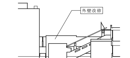
渡廊下(4)西面立面図
