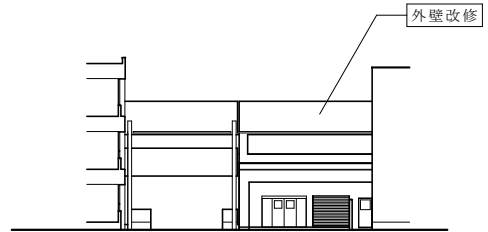
渡廊下(1)西面立面図
