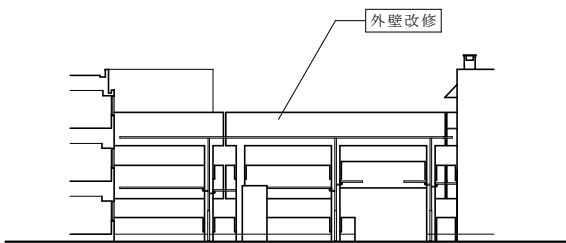
渡廊下(2)東面立面図
