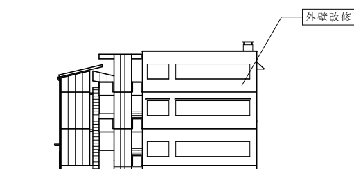
西面立面图
