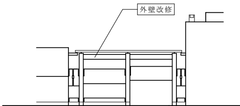
渡廊下(3)東面立面図
