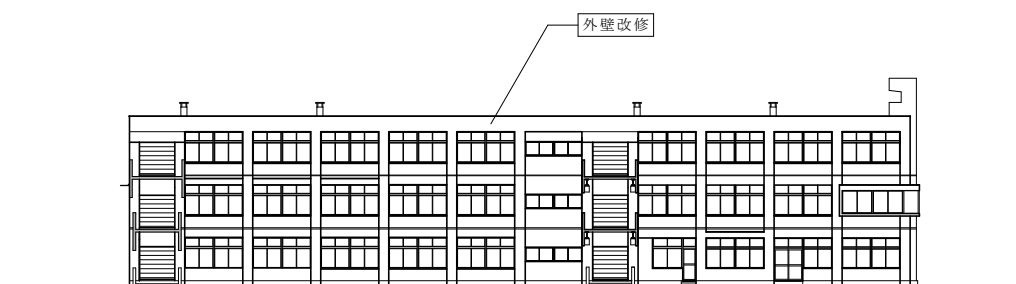
南面立面图
