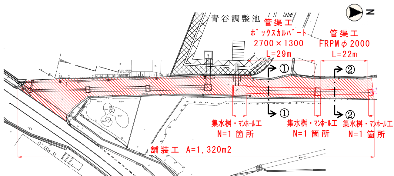
計画平面図
