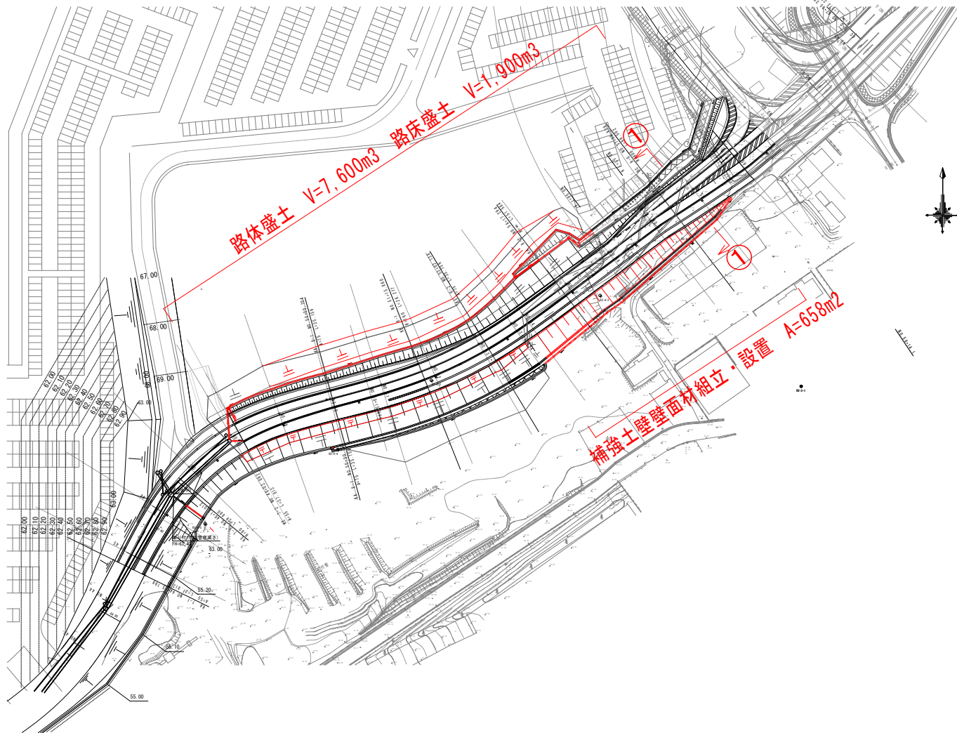
計画平面図
