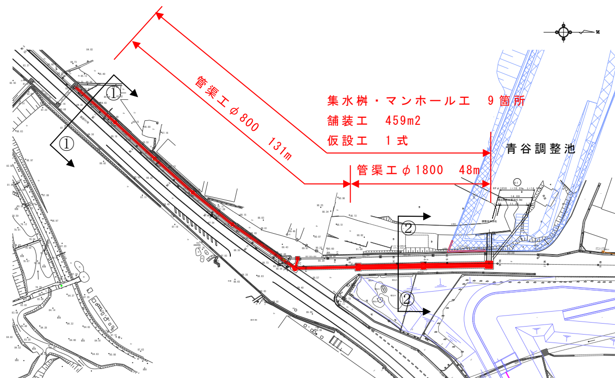
計画平面図
