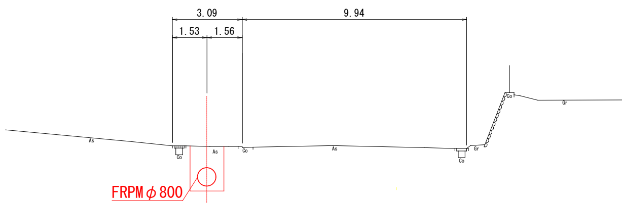
②－②断面
