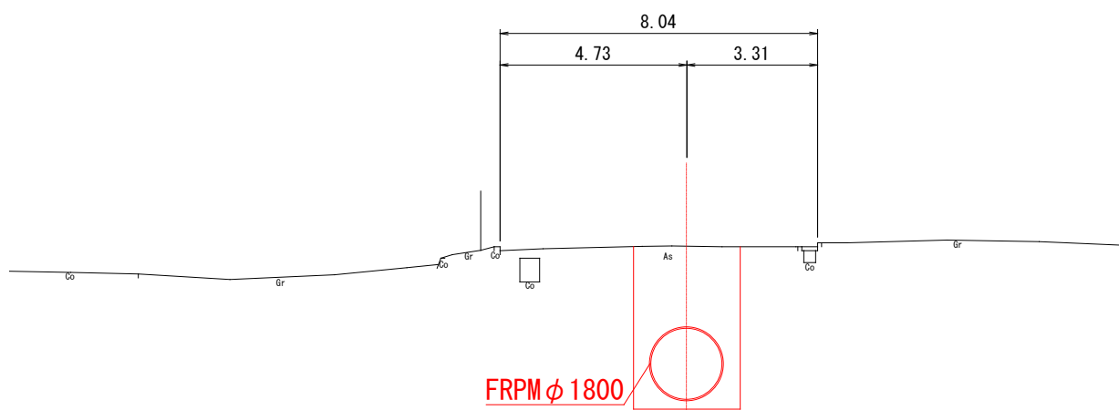
②－②断面
