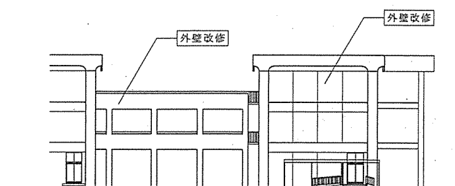
東面立面図 (渡り廊下)
