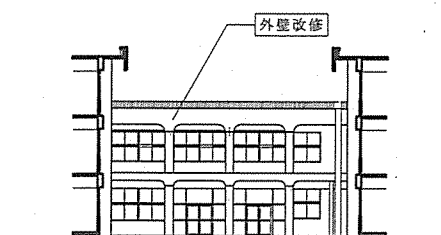
東面立面図 (1-2番棟)
