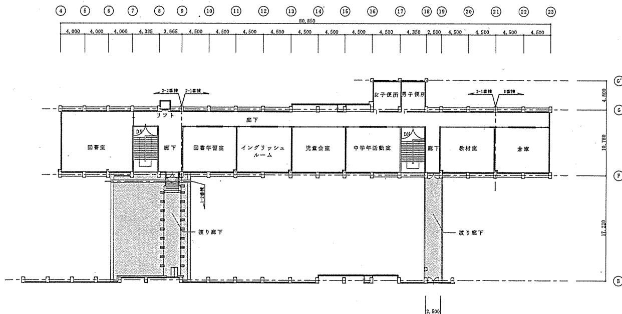
3 階平面図
