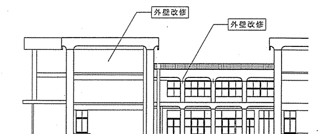
西面立面図
