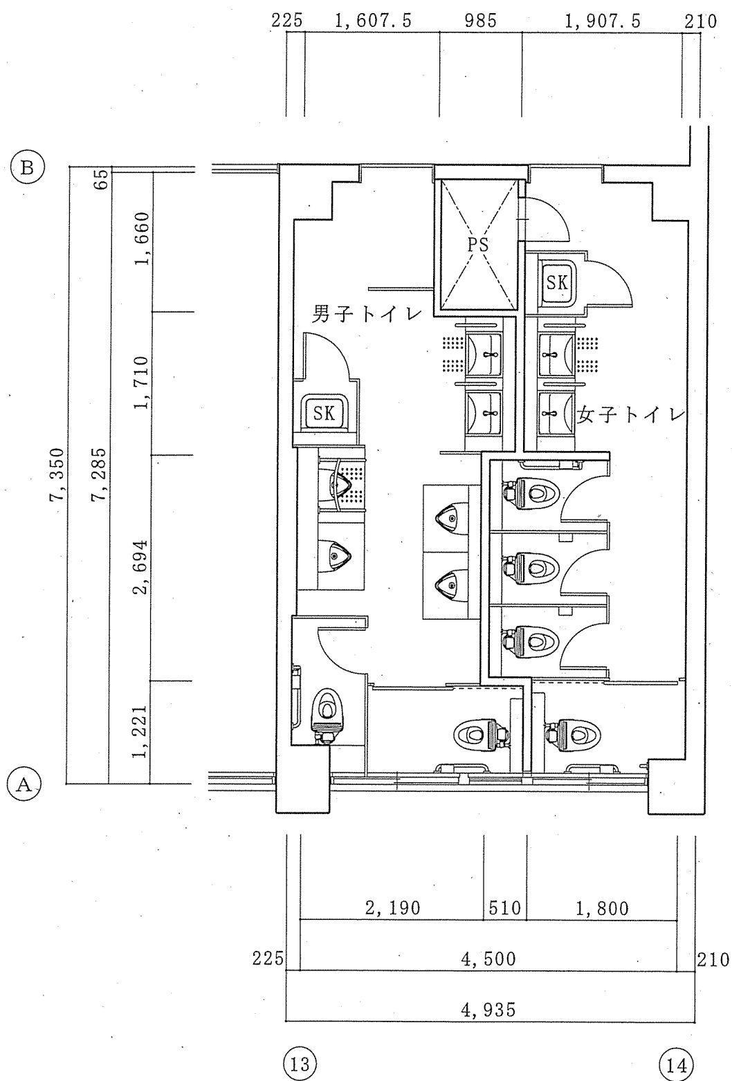
1階トイレ平面図
