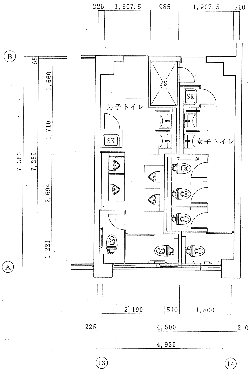
2、3階トイレ平面図
