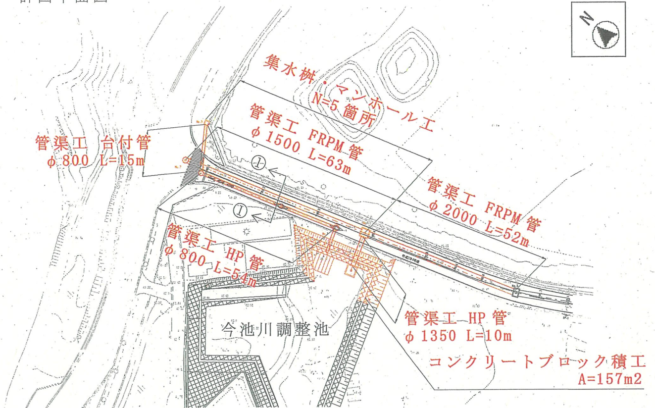
計画平面図
