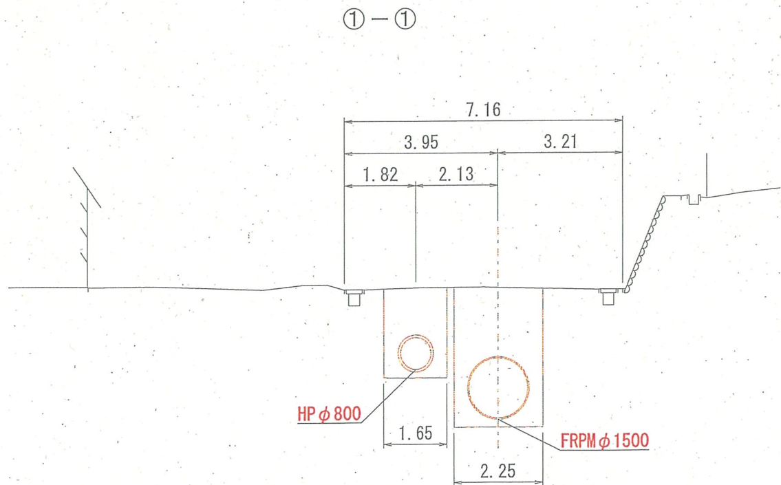
標準断面図
