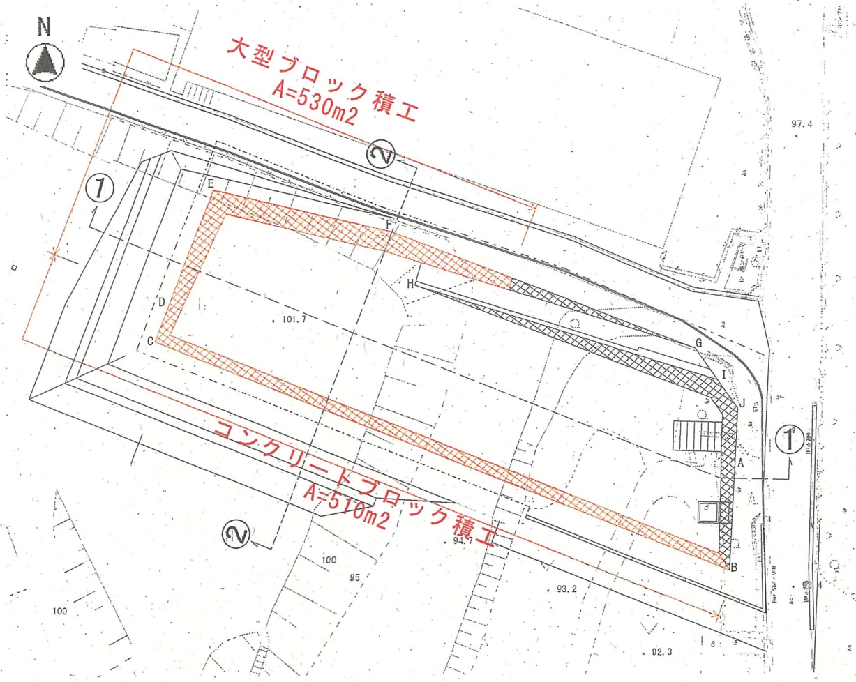
計画平面図
