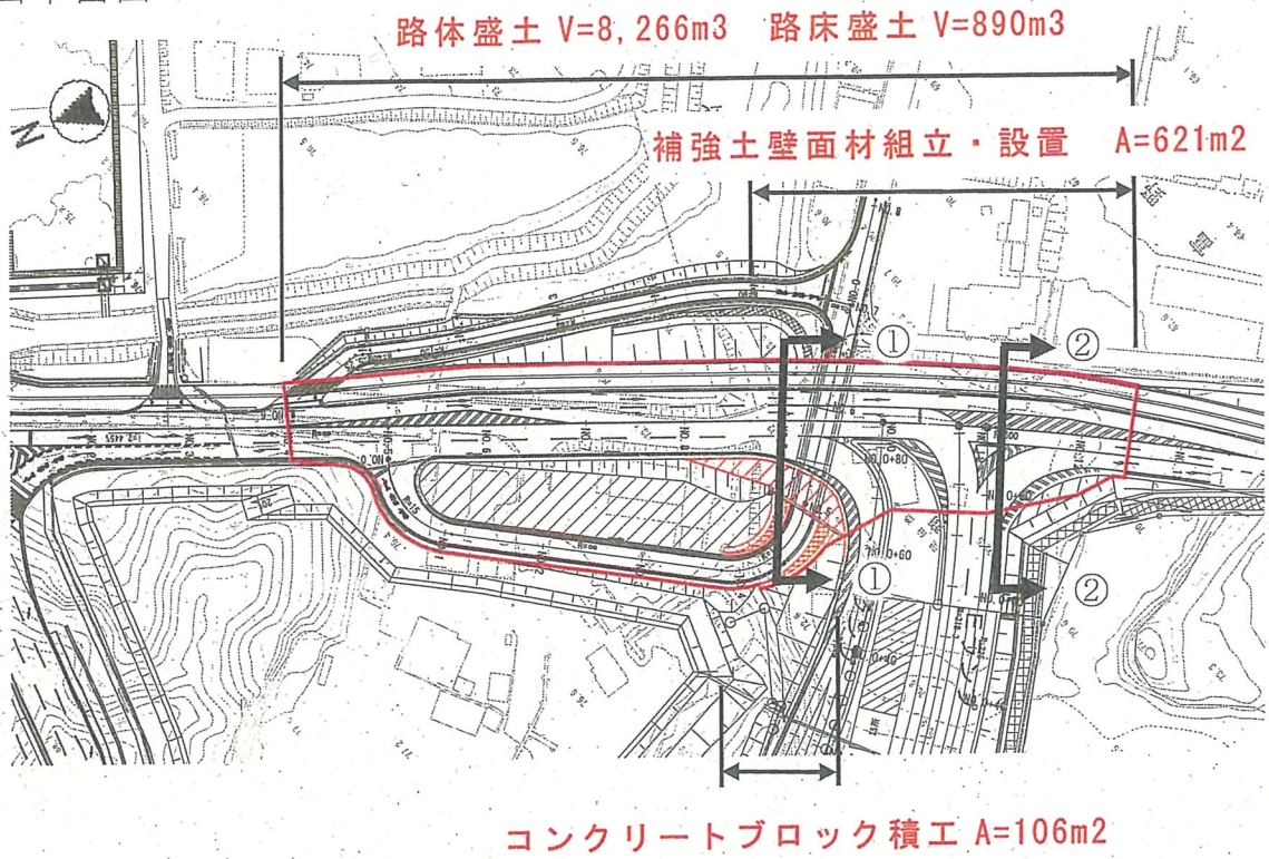
計画平面図
