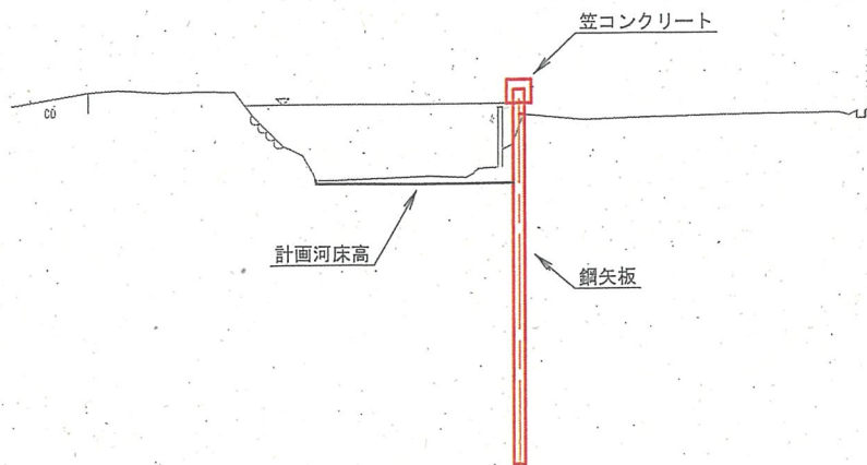
標準断面図
