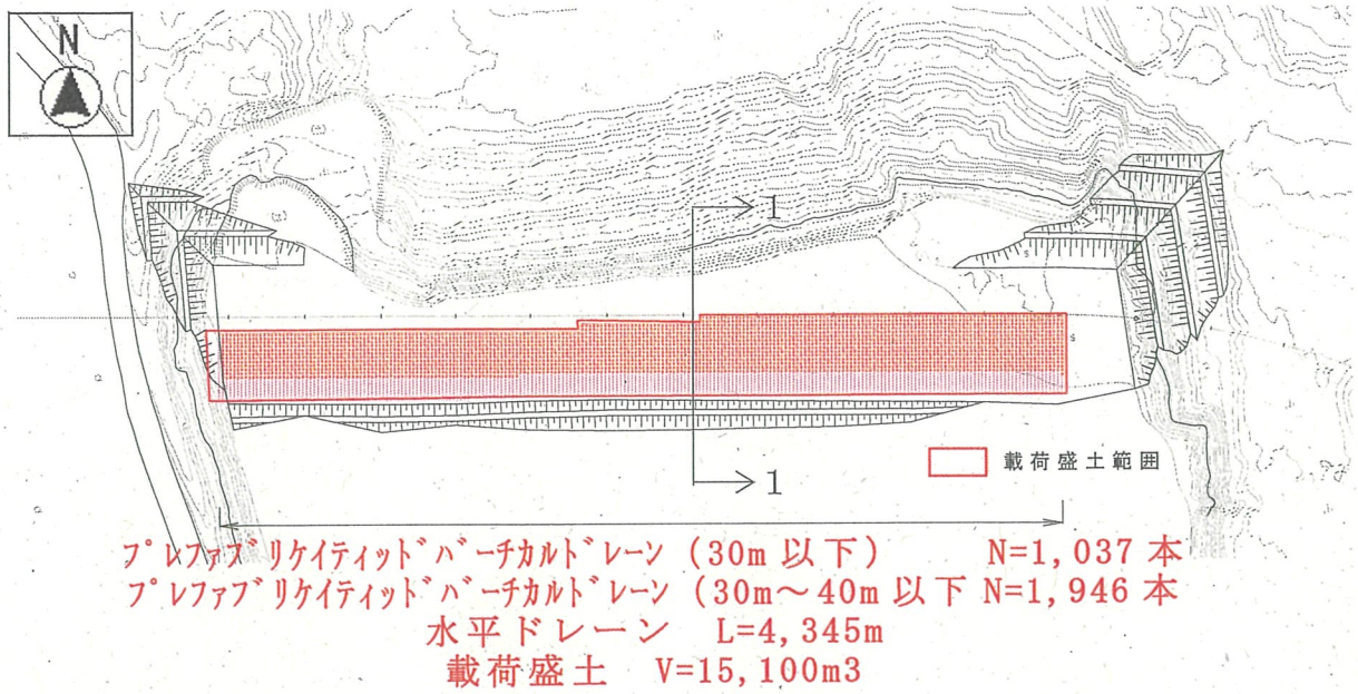
計画平面図
