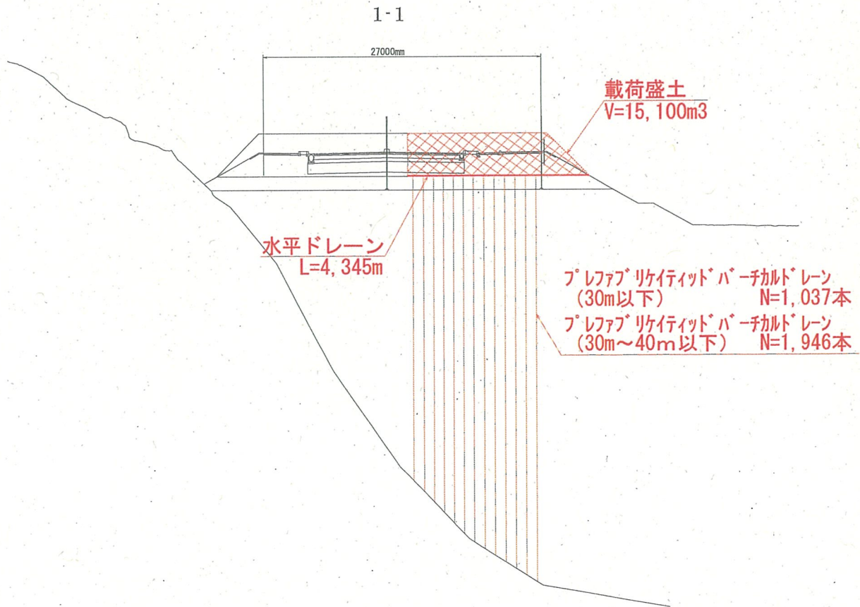
標準断面図
