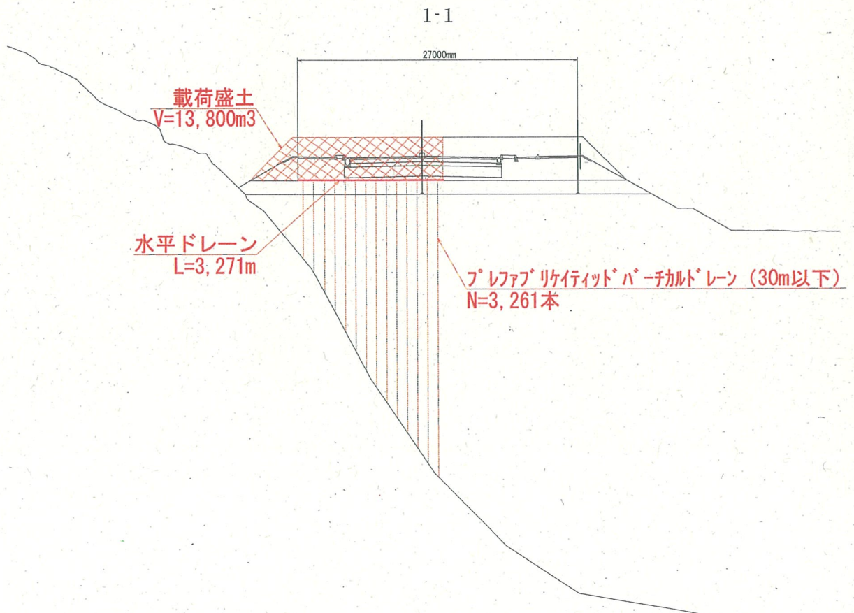
標準断面図
