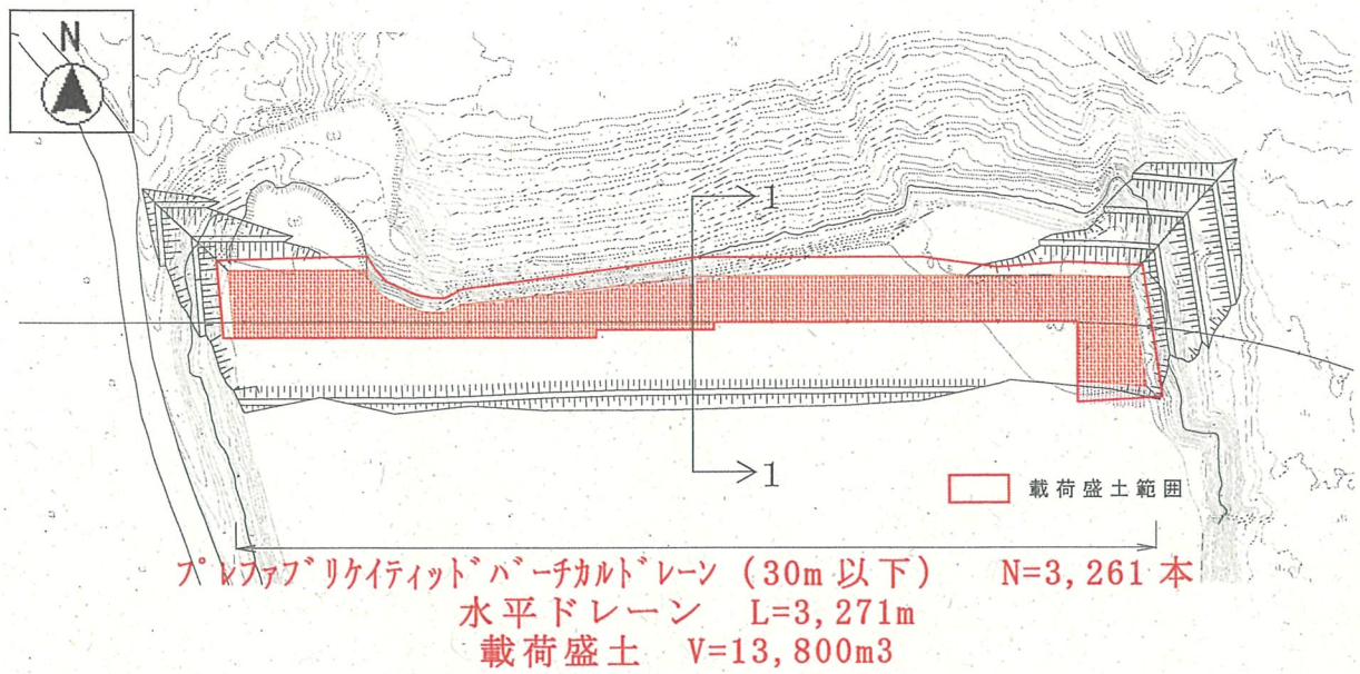
計画平面図
