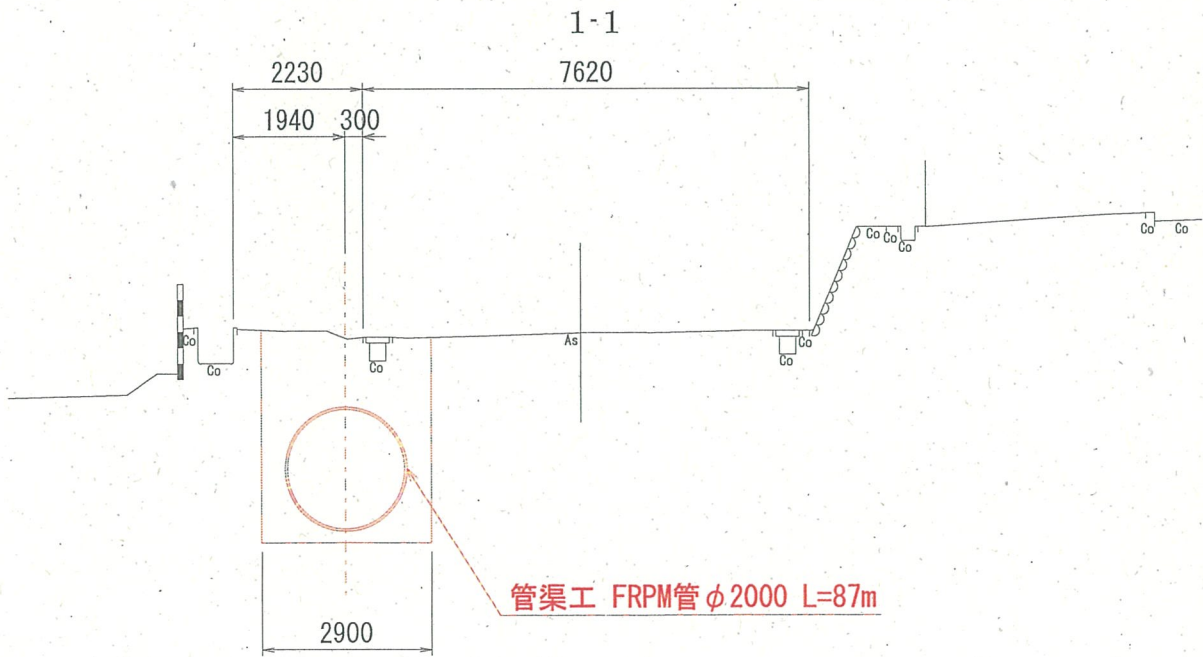
標準断面図
