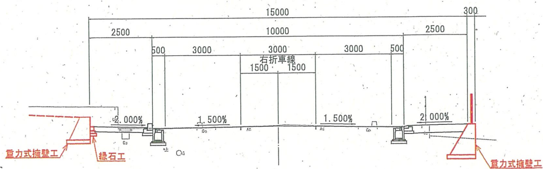
標準横断面図 A-A' s=1:100
