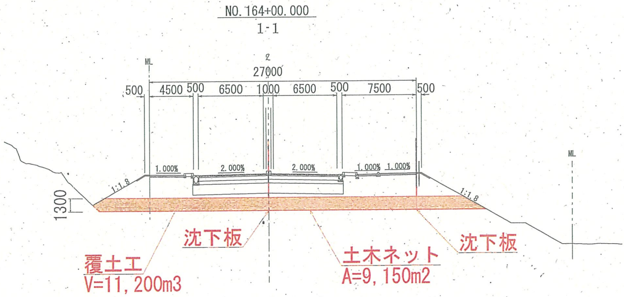
標準断面図
