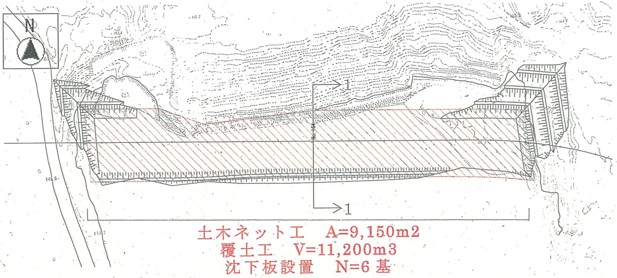
計画平面図
