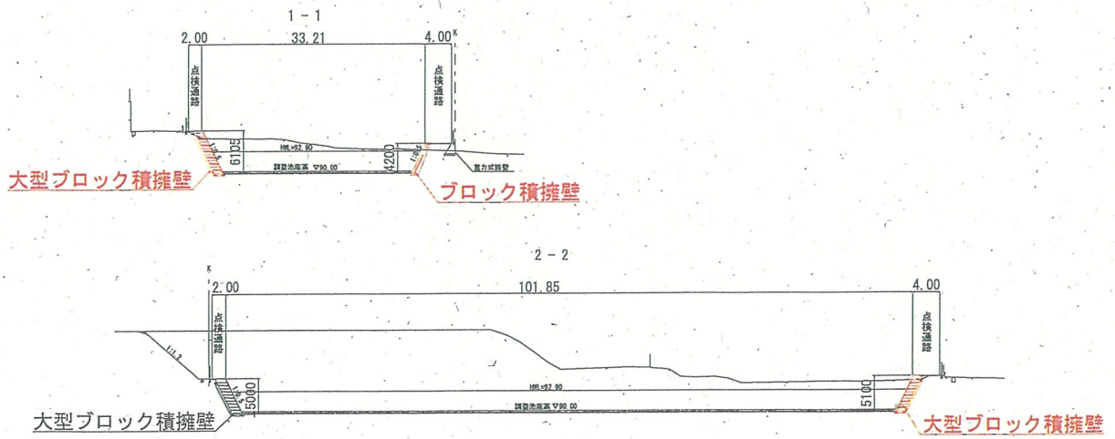
標準断面図
