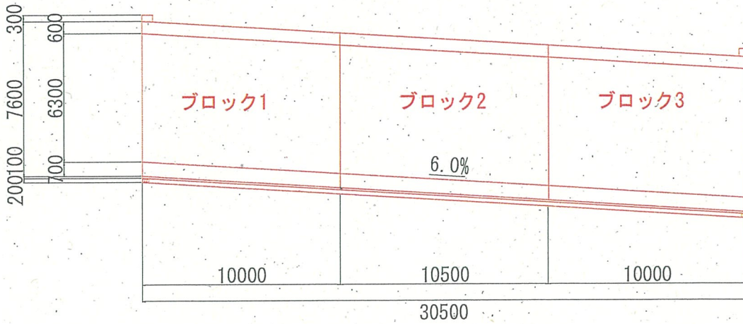
側面図
