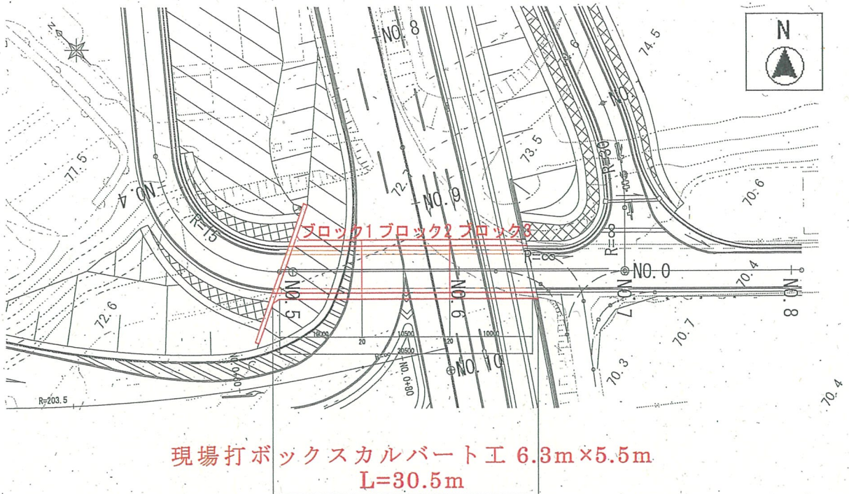
計画平面図
