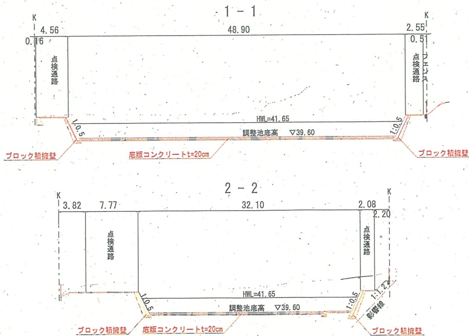
標準断面図
