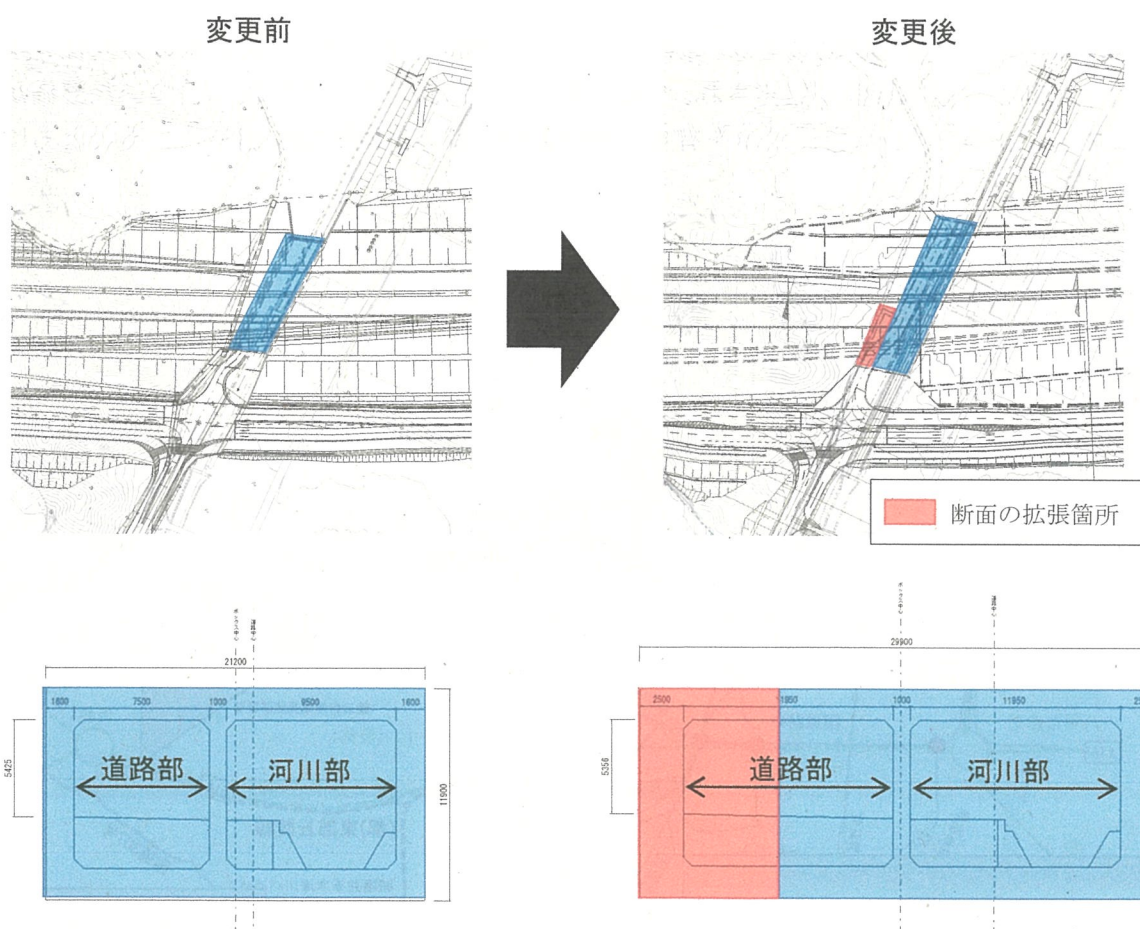
【図7 ボックスカルバート断面図】
