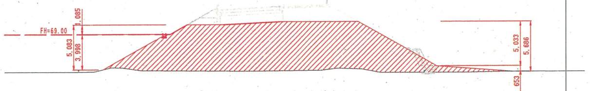
計画断面図 (B-B断面)
