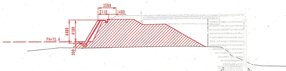
計画断面図 (C-C断面)
