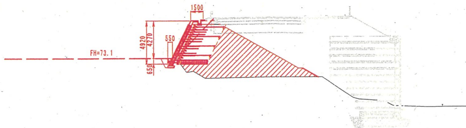
計画断面図 (C-C断面)
