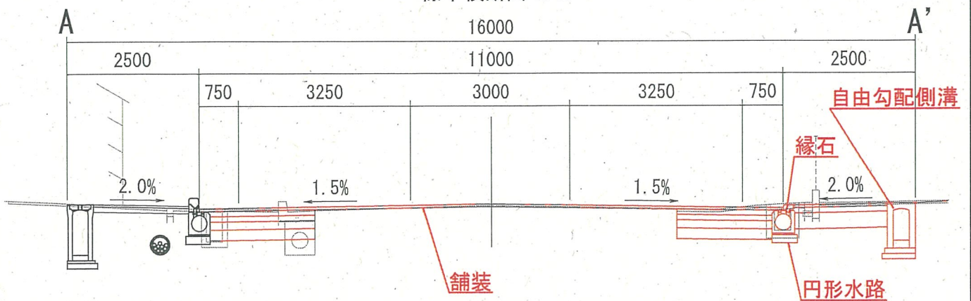
標準横断面図 A-A'
