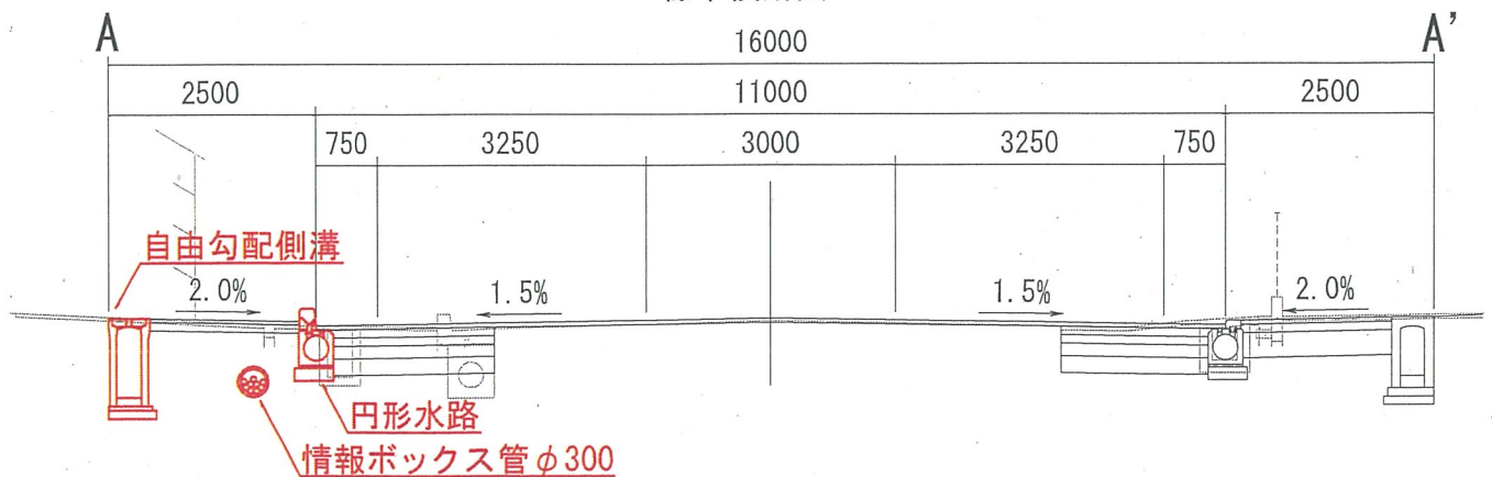
標準横断面図 A-A'
