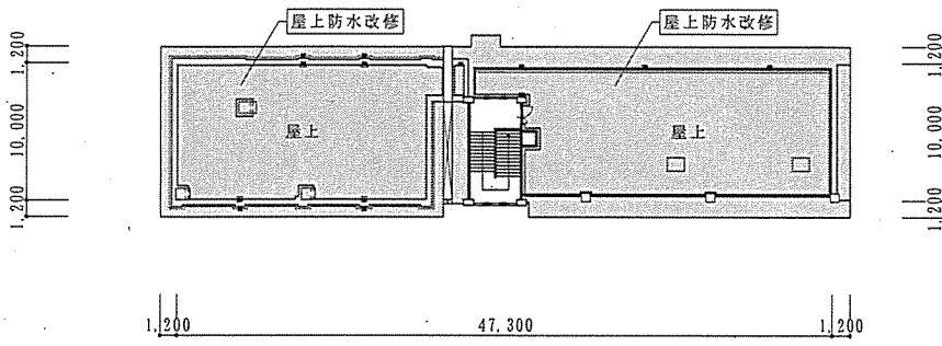
R階平面図
