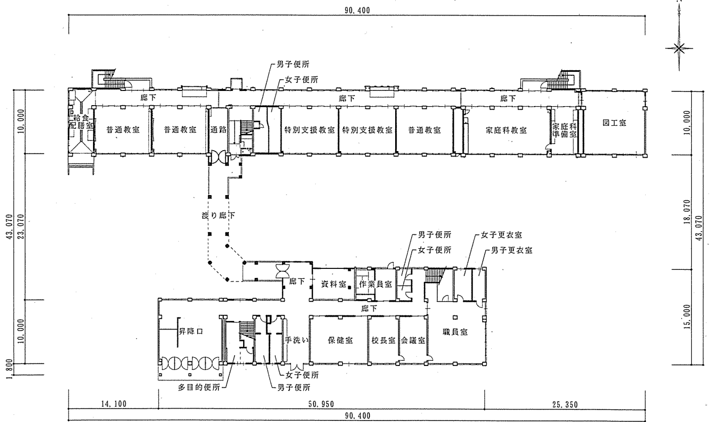
1 階 平 面 図
