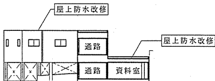
南側立面図
