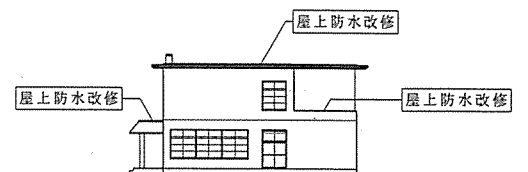
東側立面図
