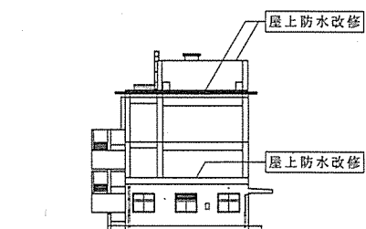
西側立面図
