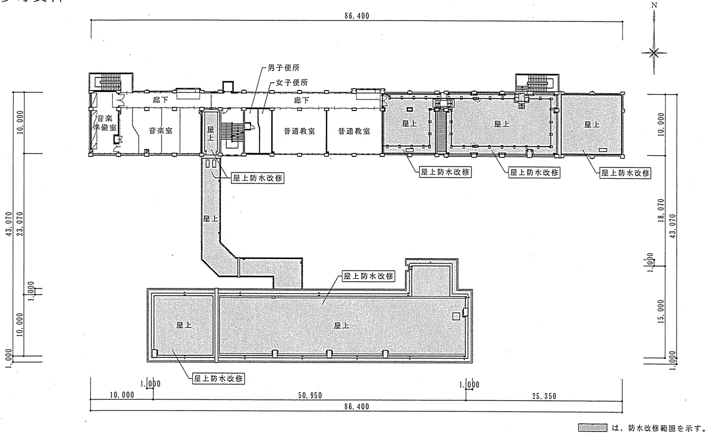
3 階 平 面 図
