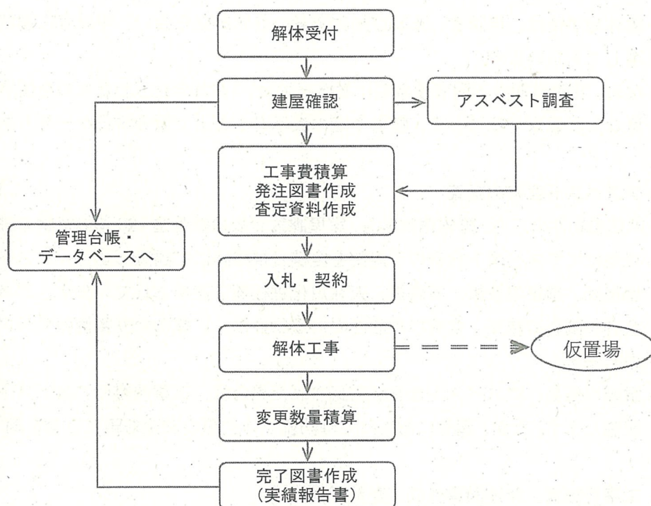
図7 家屋・建屋解体の流れ
