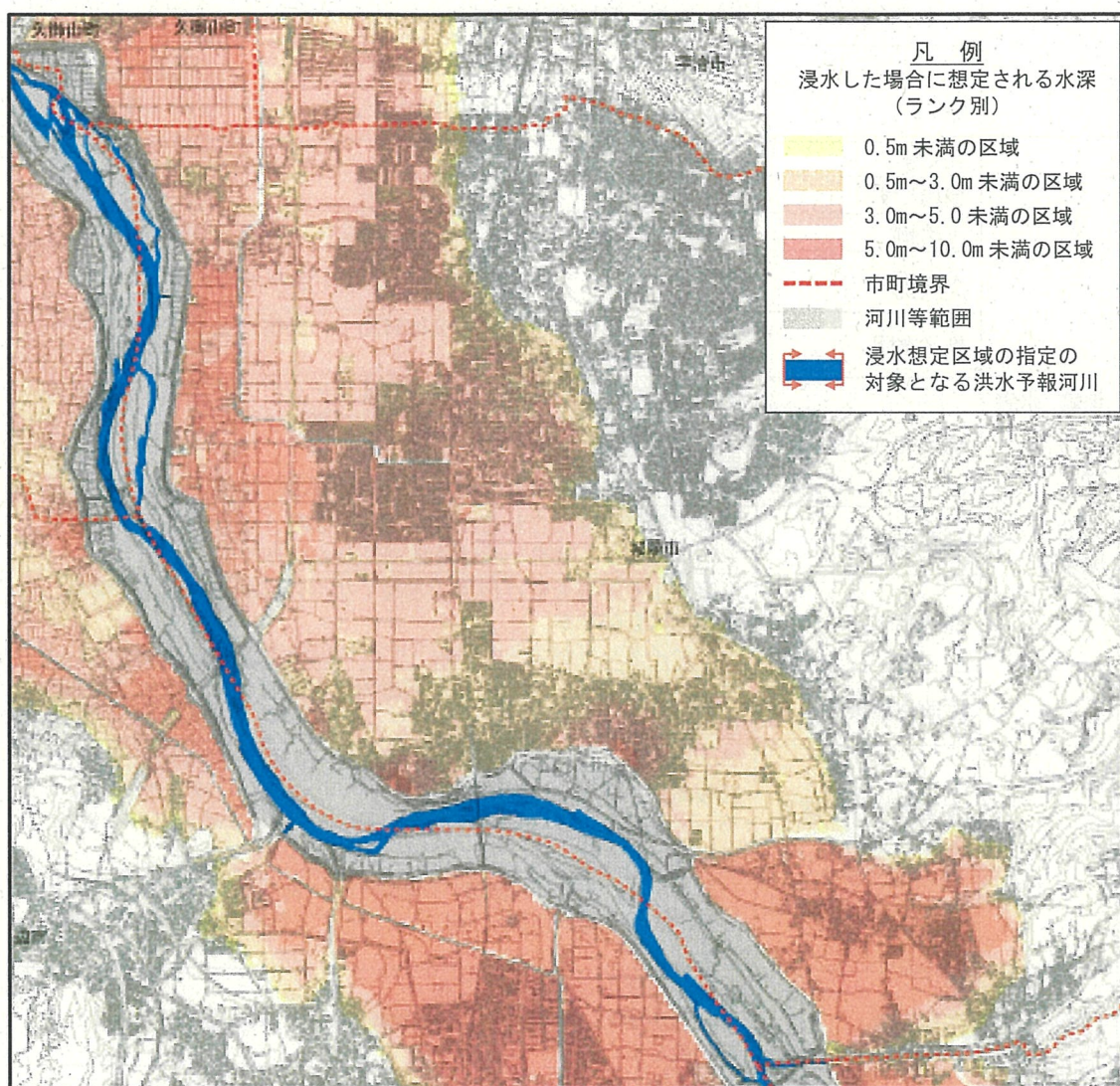
図3 洪水浸水想定区域図（想定最大規模：木津川）
