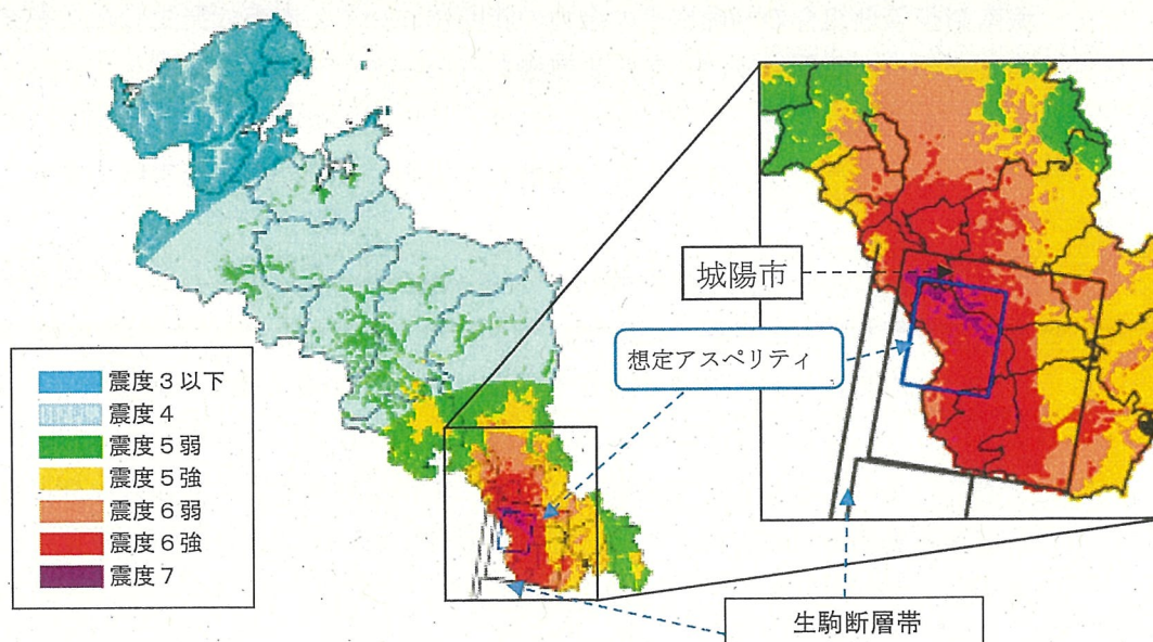
図2 生駒断層帯 震度分布図
