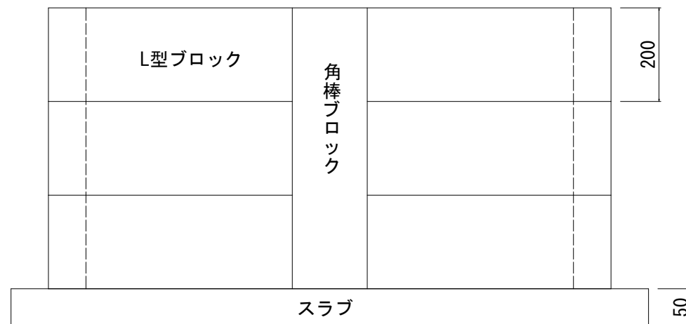
断面図
