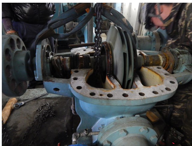
図 4-8 老朽化したポンプ
