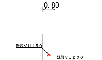
断面図 s=1:20
