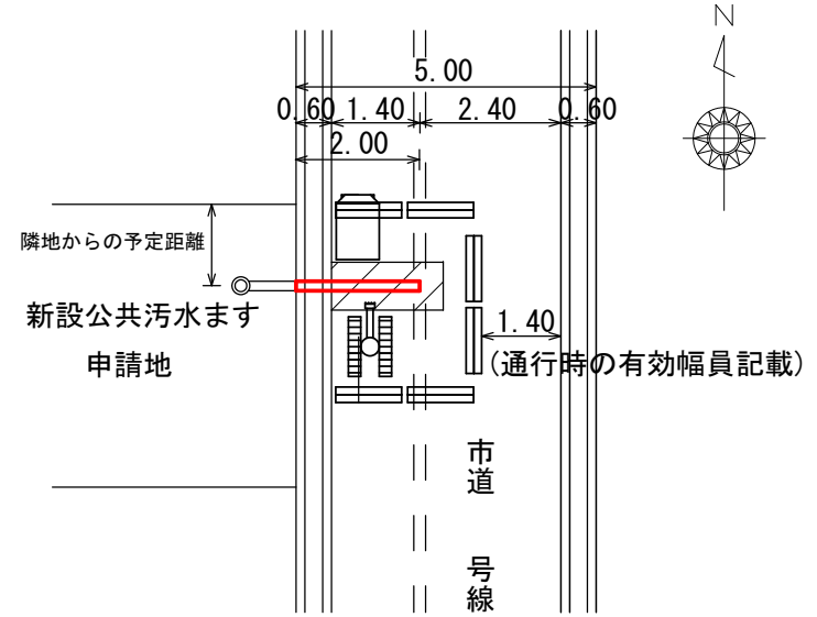
平面図 s=1:100
