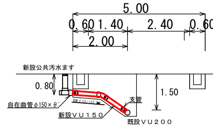
横断面図 s=1:100
